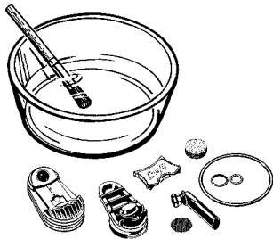
Manuelle Reinigung der zerlegten Kühleinheit
