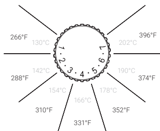
Verdampfungstemperatur-Skala
