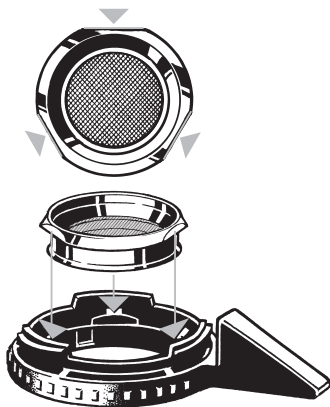
Cylindre de la Chambre de Remplissage, Boîtier de la Chambre de Remplissage, Surfaces de Positionnement
